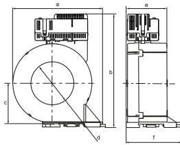
MRCDB30... + CTBC60(P)
