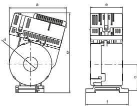
MRCDB30... + CTBC20(P)/CTBC35(P)
