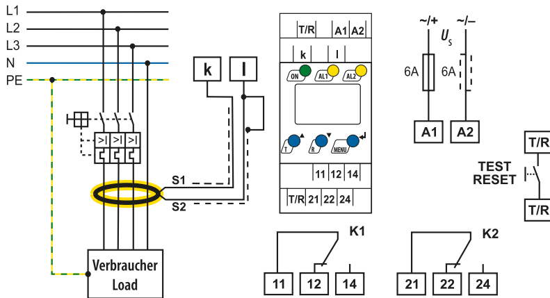
Abbildung: Anschlussbild
